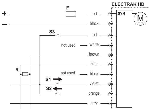
Slave actuators
